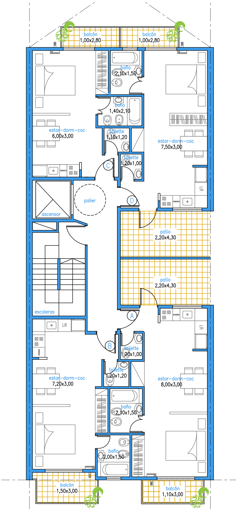
PALESTINA 528 - PLANTA 1º PISO
