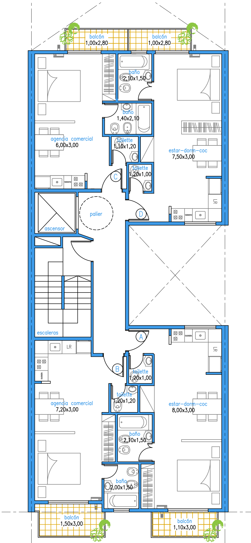
PALESTINA 528 - PLANTA TIPO 2º A 6º PISO
