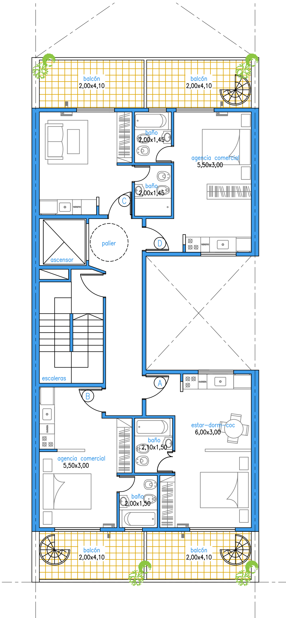
PALESTINA 528 - PLANTA 7º PISO
