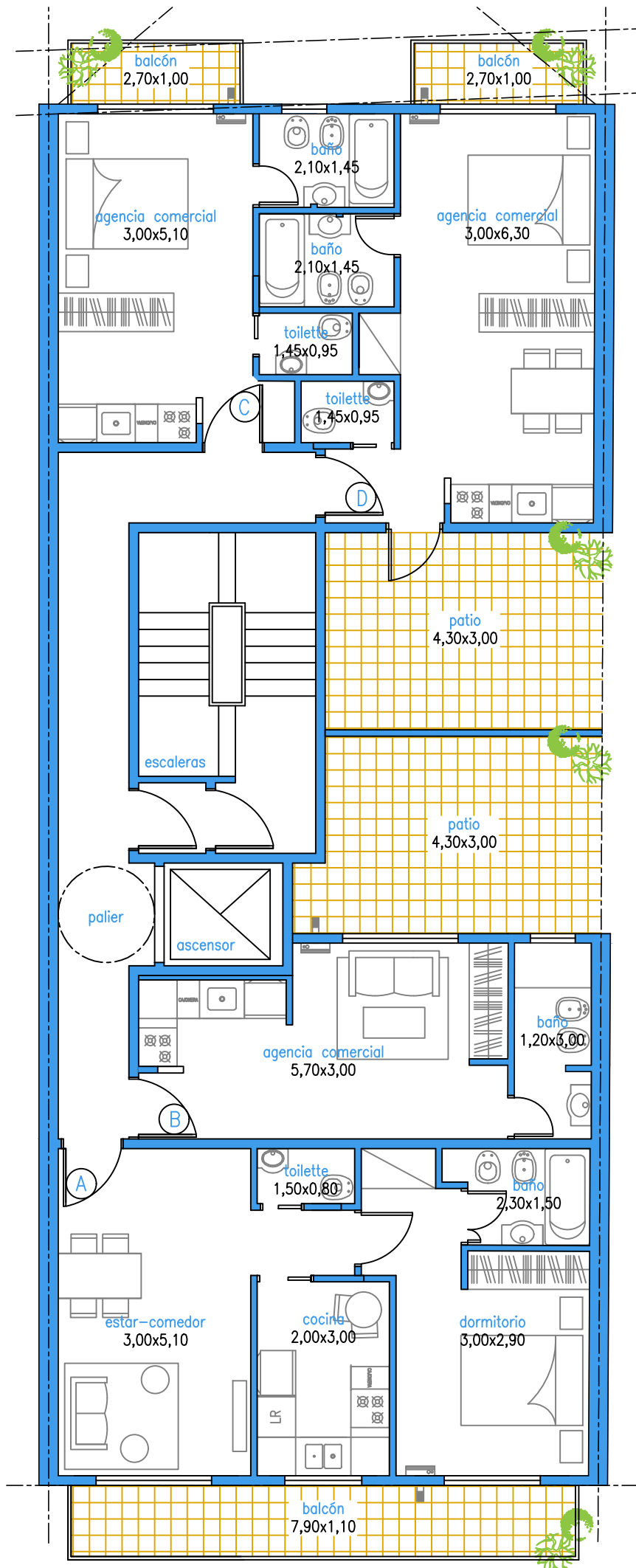
LAMBARÉ 847 - PLANTA 1º PISO
