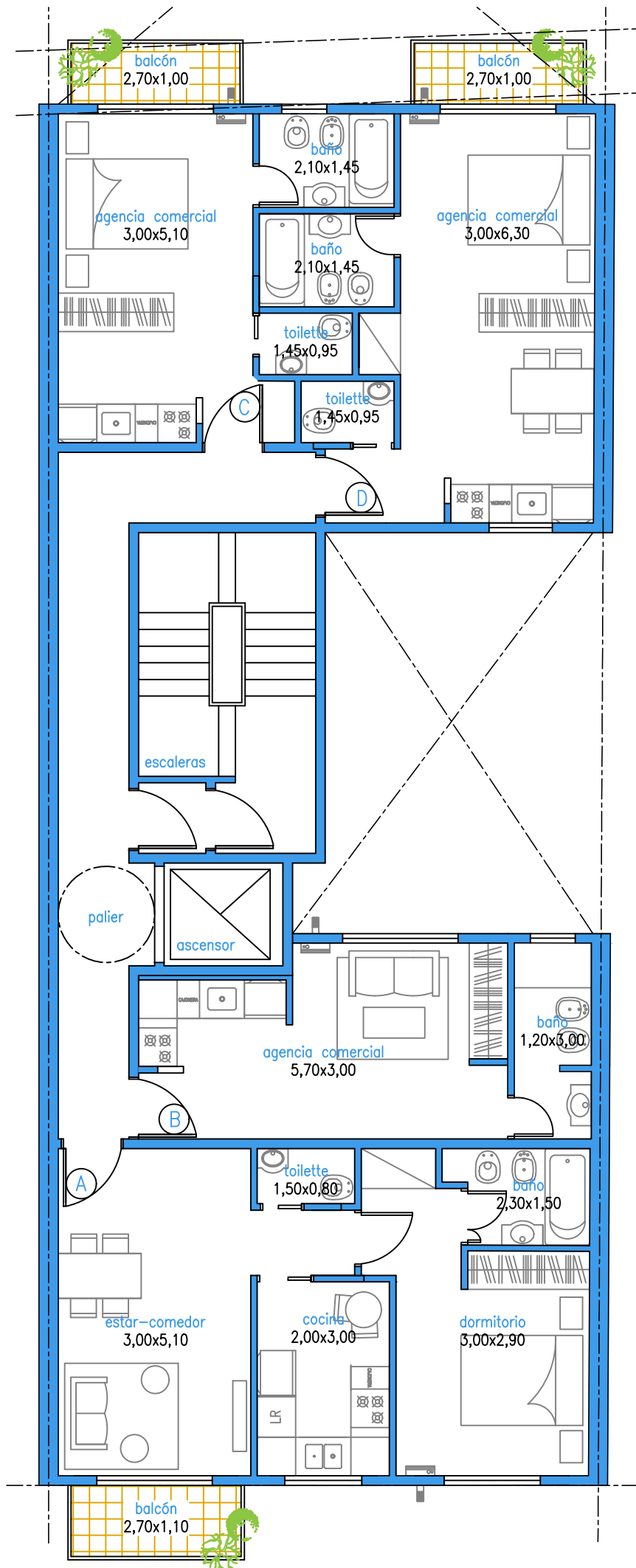
LAMBARÉ 847 - PLANTA TIPO 2º A 7º PISO
