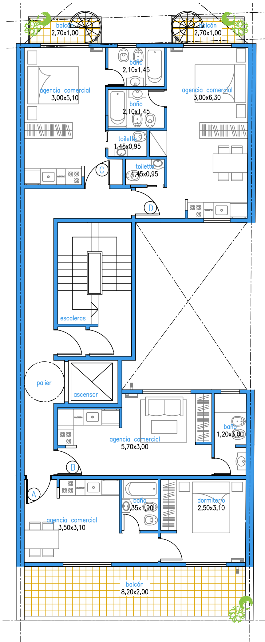
LAMBARÉ 847 - PLANTA TIPO 8 º PISO
