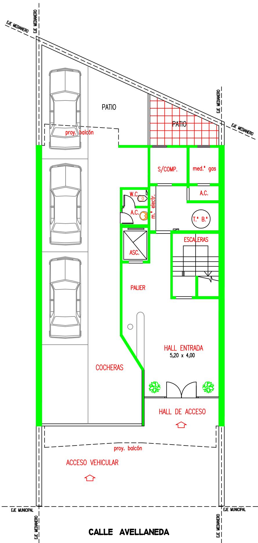
PLANTA BAJA AVELLANEDA II-13
