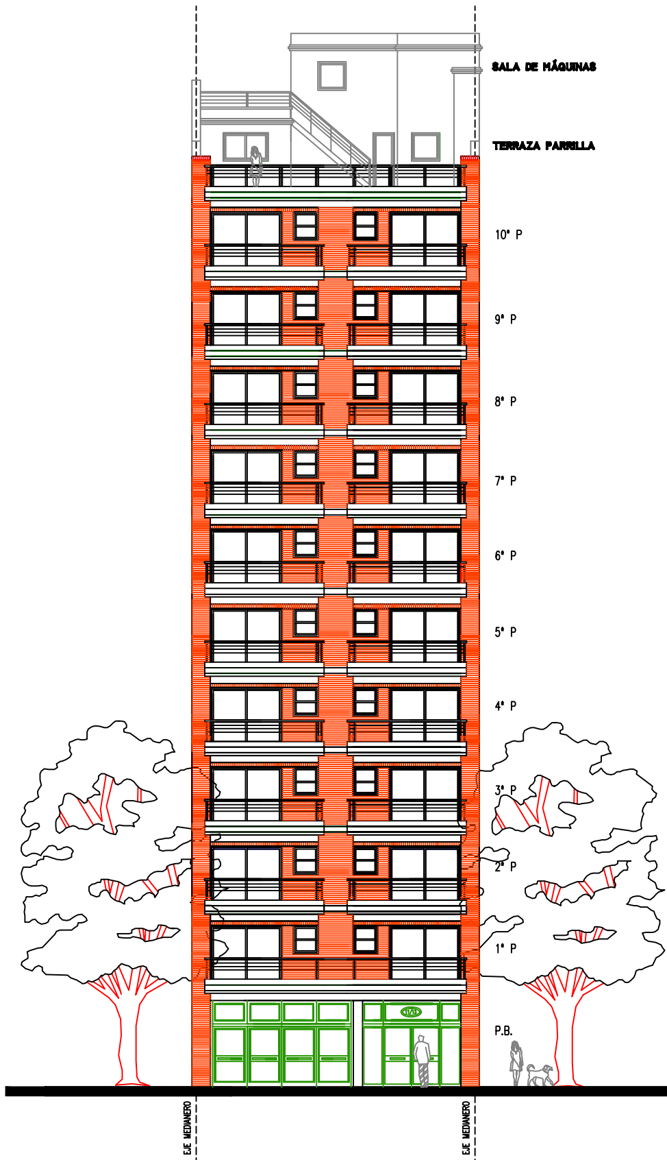
FACHADA AVELLANEDA II-13
